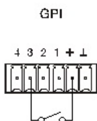
Exemple de connexion du port GPI 3
