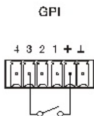
Exemple de connexion du port GPI 3
