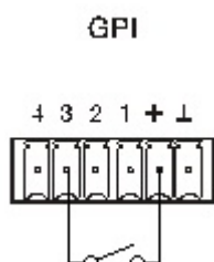
Beispiel für den Anschluss von GPI 3
